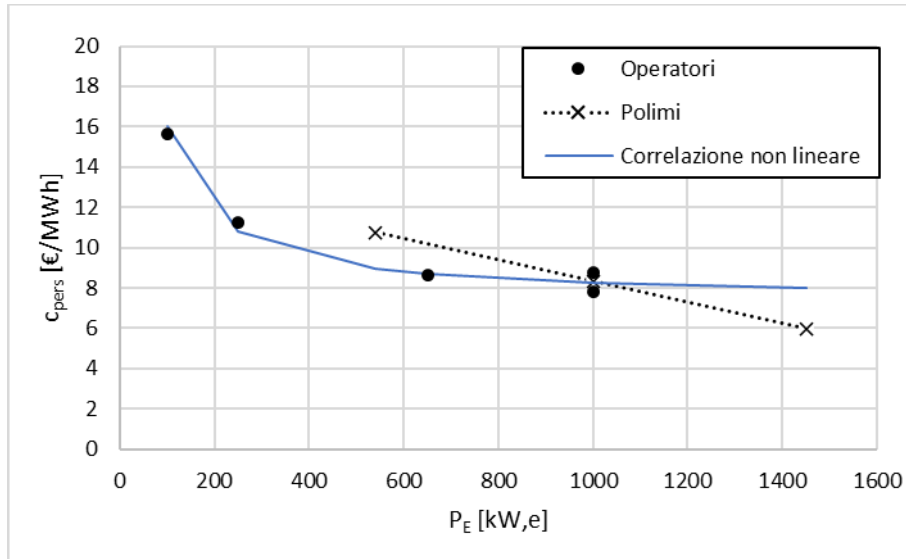
Figura 1: correlazione tra costo del personale e potenza elettrica installata
