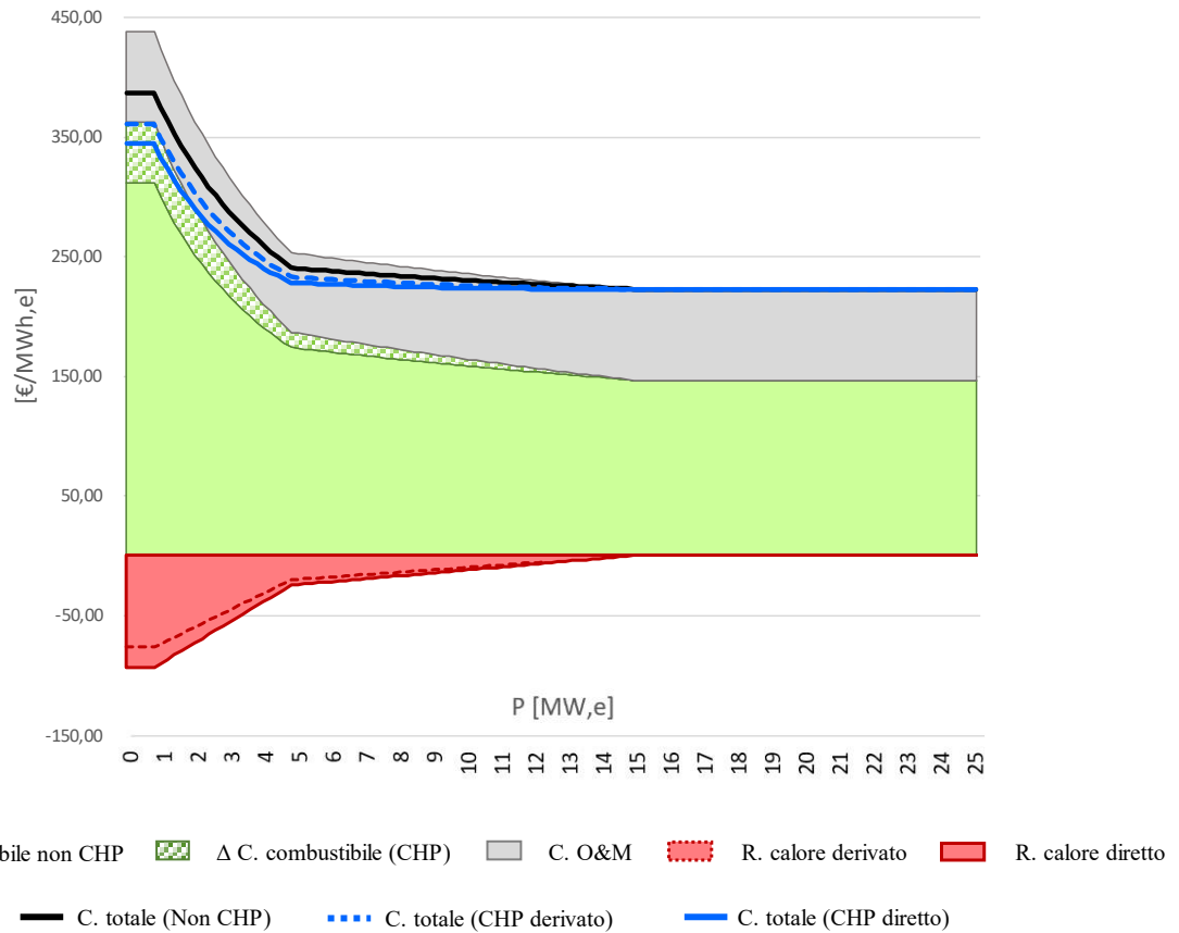
Figura 6: Andamento dei costi di generazione rispetto alla taglia dell’impianto.
