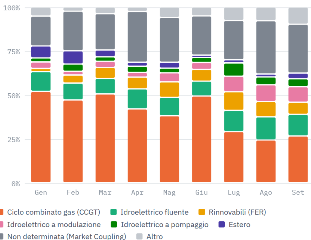
Figura 2.4a - tecnologie marginali (nel caso della voce “market coupling” e della voce “estero” la tecnologia marginale non è in Italia e non può essere univocamente identificata; la voce “altro” include le batterie elettrochimiche e gli impianti termoelettrici non alimentati da gas naturale) nel periodo gennaio-settembre 2026
