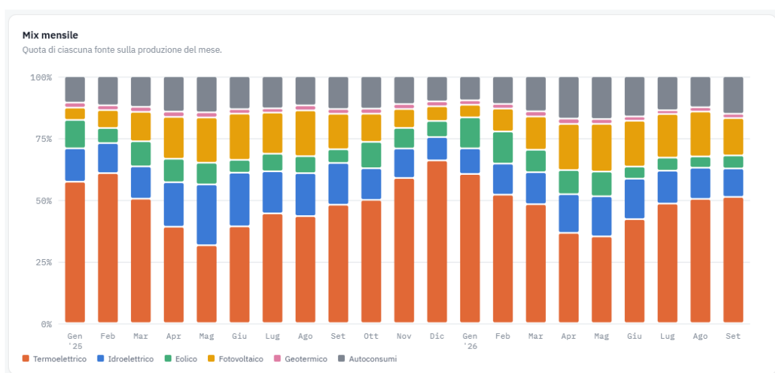
Figura 3.3b - Quota mensile per tecnologia nel periodo gennaio 2025 – settembre 2026
