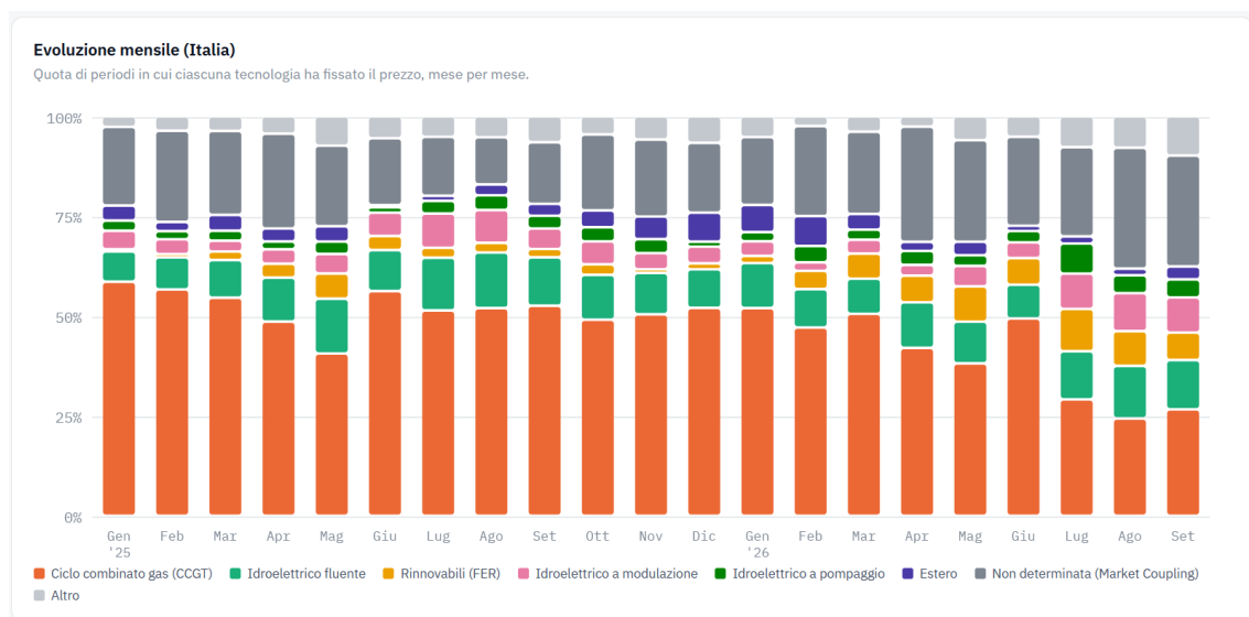
Figura 2.4b - tecnologie marginali (nel caso della voce “market coupling” e della voce “estero” la tecnologia marginale non è in Italia e non può essere univocamente identificata; la voce “altro” include le batterie elettrochimiche e gli impianti termoelettrici non alimentati da gas naturale) nel periodo gennaio 2025-settembre 2026
