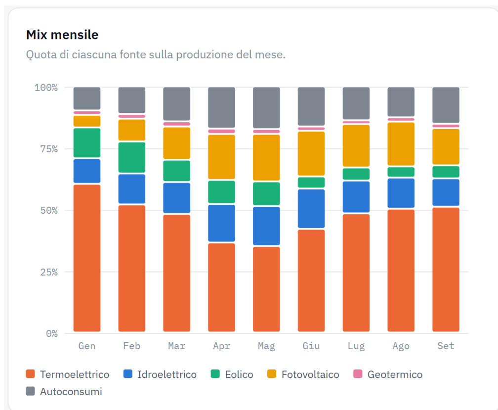
Figura 2.3a - Quota mensile per tecnologia nel periodo gennaio – settembre 2026
