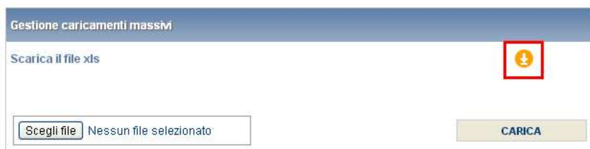
Figura 3.5: Caricamento massivo
